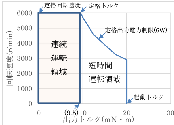
モータの運転領域 (SL22R, A1-SL22R 共通)
