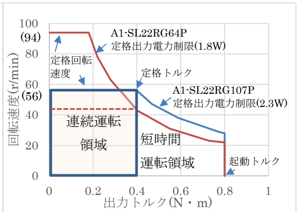
ギアモータ運転領域
